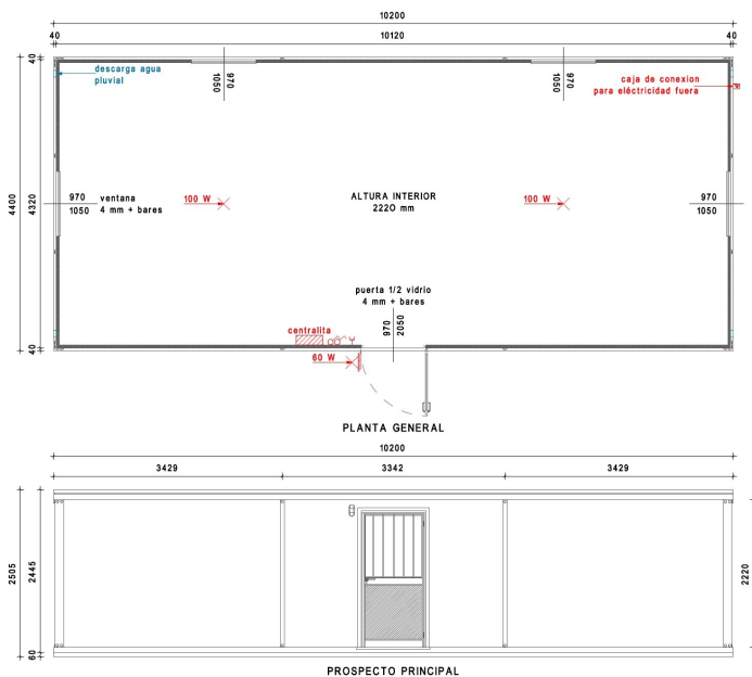
Configuración Monobloque 10200x4400
