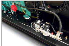
Dispositivo rabbocco automatico serbatoio Automatic refueling device Dispositif remplissage automatique Recarga automática de combustible
