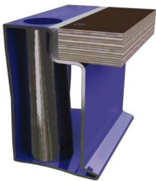
Profilo Brevettato T20962 Acciaio UNI EN 1002 - S275JH01 Perfil Patentado de Acero T20962 UNI EN 10025 - S275JH01 Patented Steel Profile T20962 UNI EN 10025 - S275JH01
